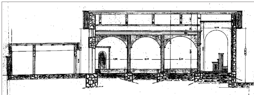
Fig. 29 Sezione trasversale: anno 2001
