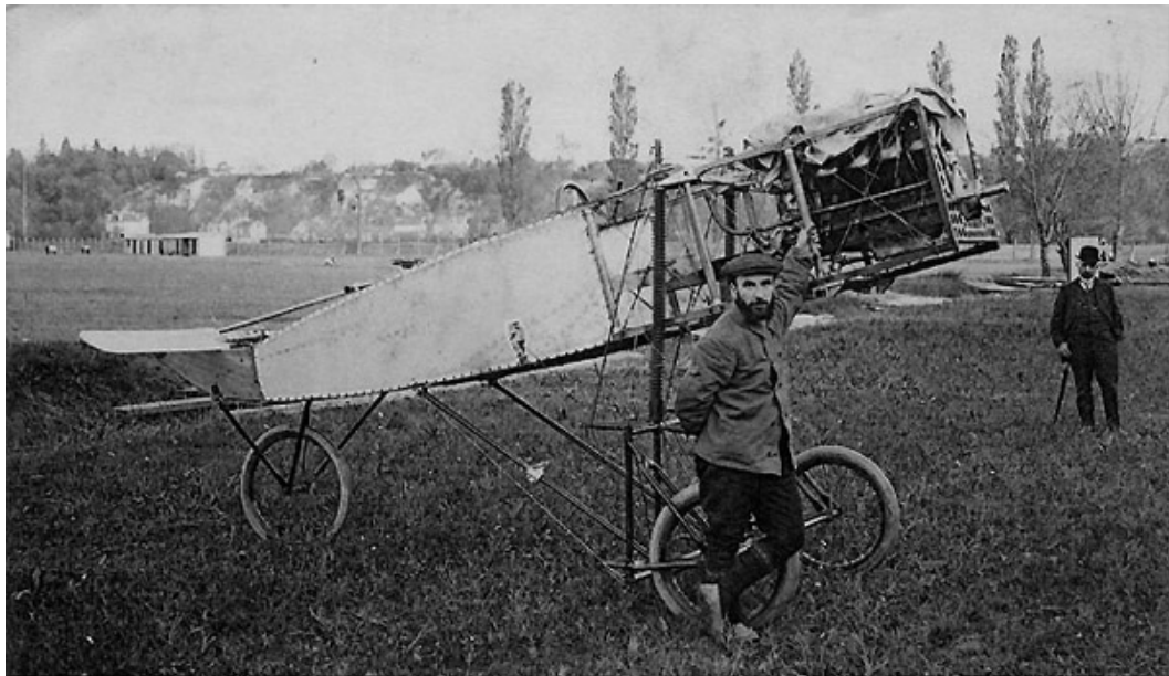
SEMAINE D'AVIATION DE TOURAINE (30 avril - 5 mai 1910). — Édition officielle. (ND Phot.) 37 — CHAMPEL et le fuselage de son biplan Voisin, 10 m. d'envergure; moteur E.N.V. de 55 HP.
