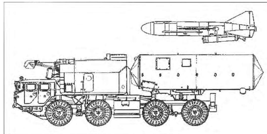
Neuvostoliitossa Styxistä rakennettiin myös rannikkoversio. Lavetilla oli kaksi ohjusta ja oma maalinsoitustutka.
